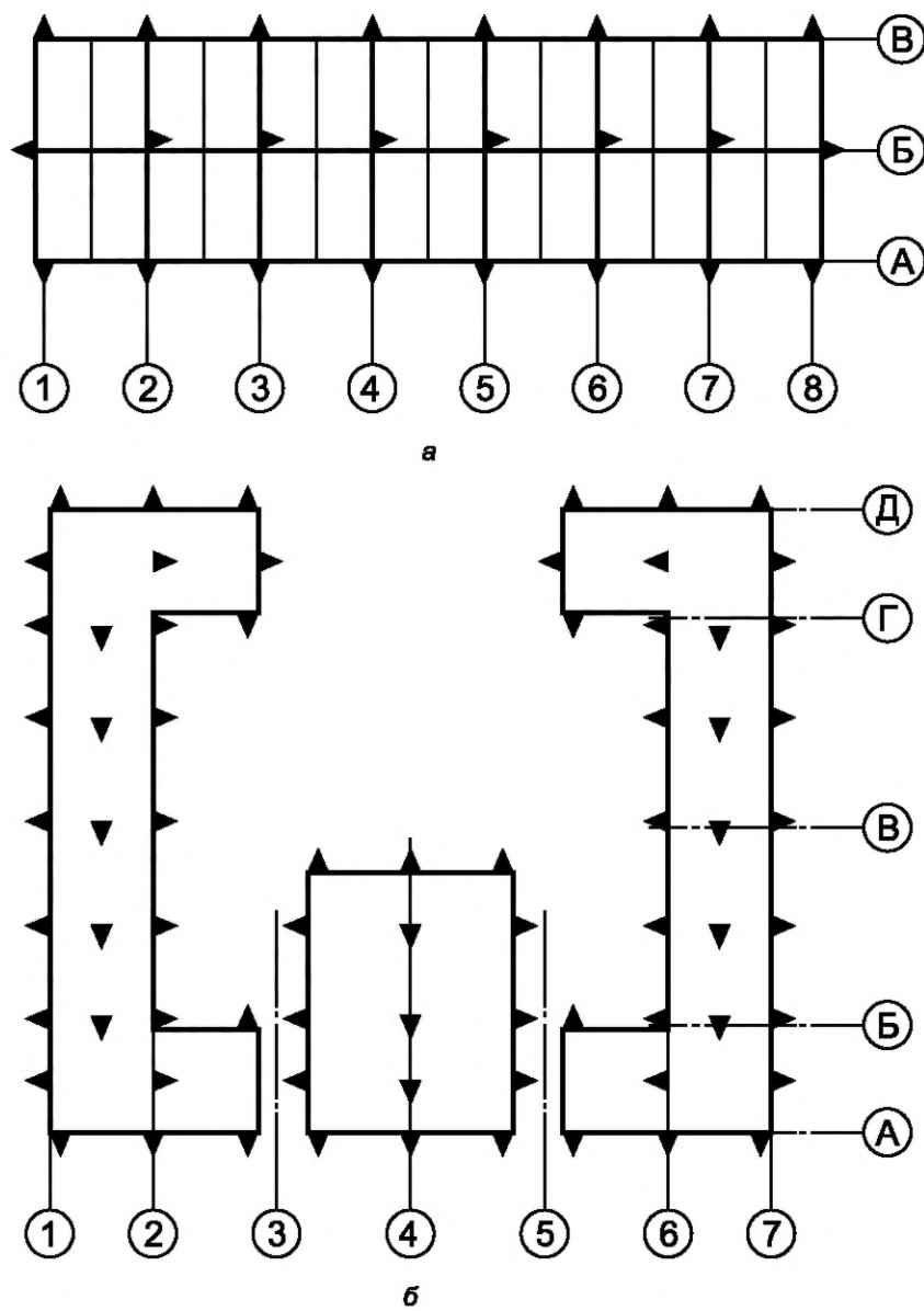
Рисунок А.1 — Схемы расположения деформационных марок на жилом доме (а) и административном здании (б)
