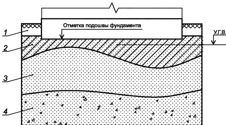
Рисунок Б.1 — Схема фундамента и основания
